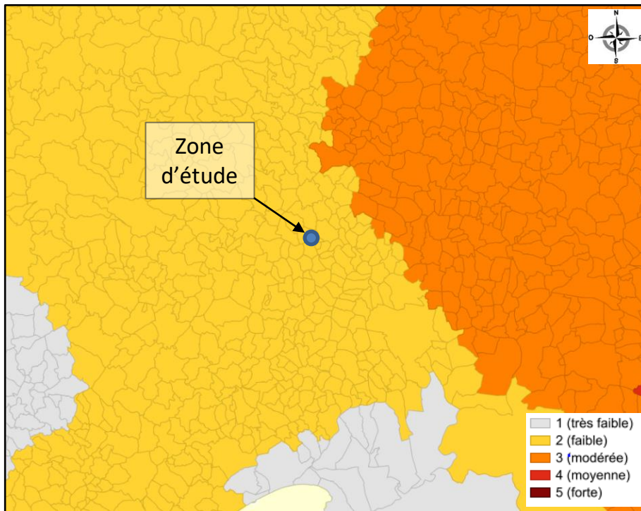
Figure : Extrait de la carte de sismicité de la commune de RIBaute LES TAVERNES (30720).
